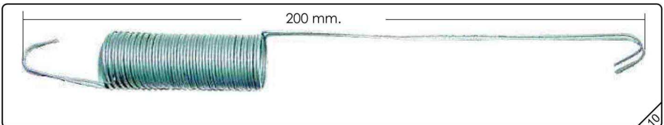
A-18 RETORNO ACELERADOR DOBLE C-35 LARGO
